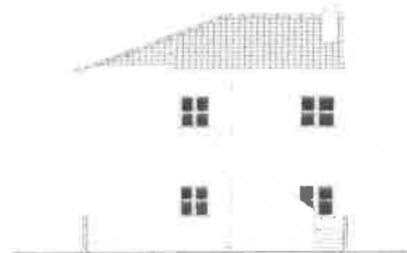
ALÇADO POSTERIOR
